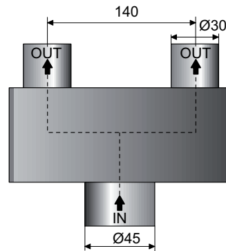
Typ 2x30 mm/1x45 mm Art.-No. 1110532 Parní výkon max. 30 kg/hod
