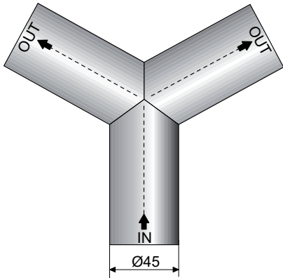
Typ 3x45 mm Art.-No. 1101164 Parní výkon max. 45 kg/hod
